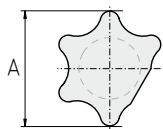
TAMPONE DI CONTROLLO PER IMPRONTA TORX (*) PLUG GAUGE FOR TORX MARK (*)
