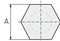
TAMPONE DI CONTROLLO PER IMPRONTA ESAGONALE PLUG GAUGE FOR HEXAGONAL MARK
